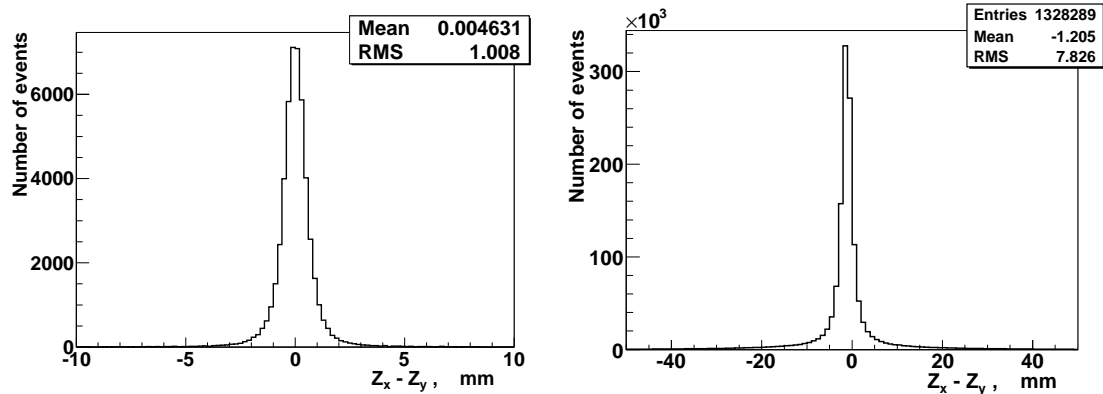
Рис. 4.14 Распределение неопределённости восстановления вершины по двум проекциям Z_x - Z_y , где Z_x — координата положения вершины в водородной мишени вдоль пучка для X-проекции, Z_y — для Y-проекции. Рисунок слева - моделированные значения, рисунок справа - экспериментальные значения неопределённостей.
