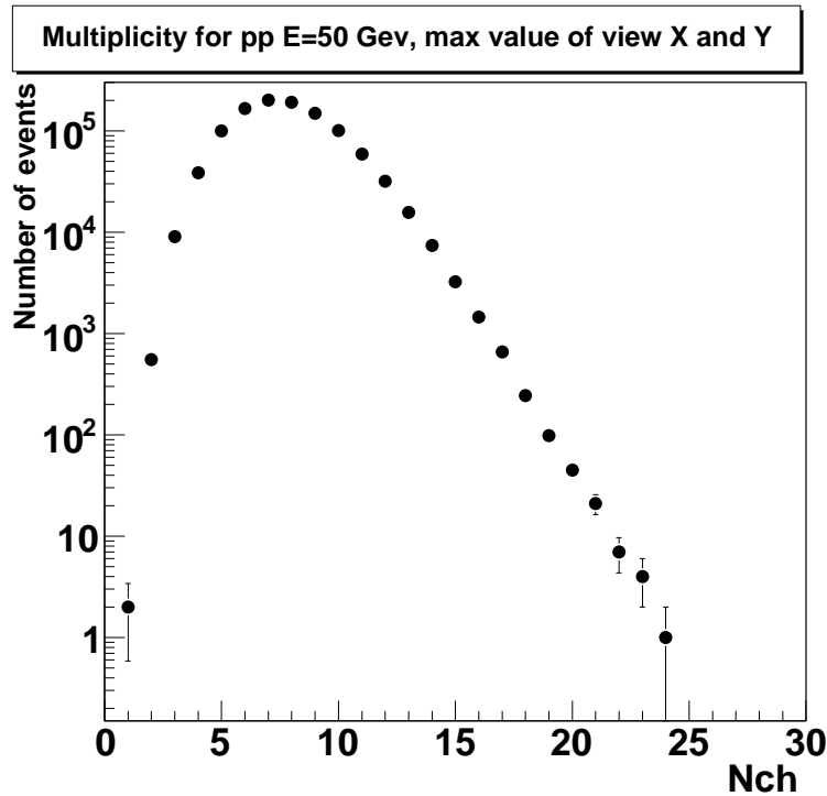
Рис. 4.35 Распределение по множественности для максимальных значений множественности на проекциях X и Y в событии, уровень триггера = 8.
