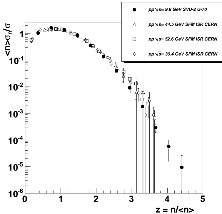
Рис. 5.5 Распределение КНО для разных энергий первичных частиц в сравнении с экспериментальными данными "Термализации". Черные кружки — данные "Термализации" для \sqrt{s} = 9.8 ГэВ полученные на SVD-2, У-70; белые ромбики, треугольники и квадраты — данные для \sqrt{s} = 30.4 ГэВ, \sqrt{s} = 44.5 ГэВ, \sqrt{s} = 52.6 ГэВ соответственно, полученные на детекторе SFM ускорителя ISR в CERN.
