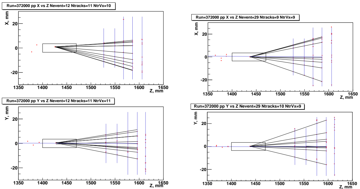
Рис. 3.32 Примеры реконструкции событий экспериментальных данных ранга 372 для 2008 года. До водородной мишени показаны хиты первичного трека в пучковом телескопе (в сжатом масштабе), а также линия трека по этим хитам, если число хитов на треке не менее трёх.
