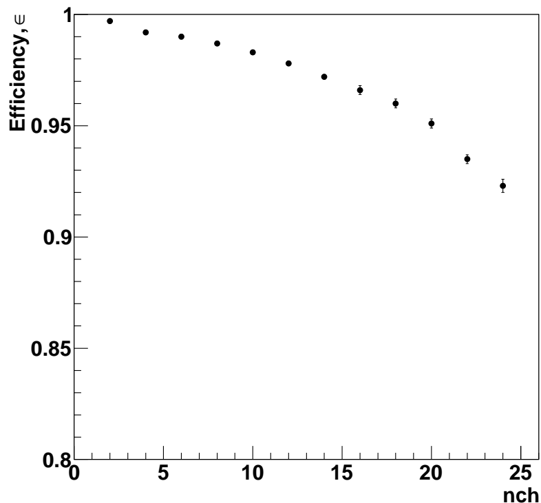
Рис. 3.37 Распределение эффективности распознавания треков от множественности по моделированным данным.
