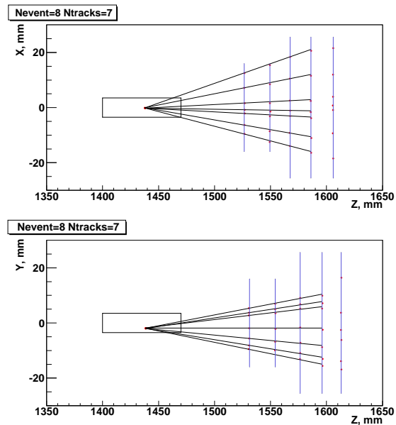
Рис. 3.31 Пример реконструкции моделированного события в вершинном детекторе. Прямоугольный бокс на рисунке — водородная мишень, вертикальные линии — детектирующие плоскости вершинного детектора, точки на плоскостях — хиты.
