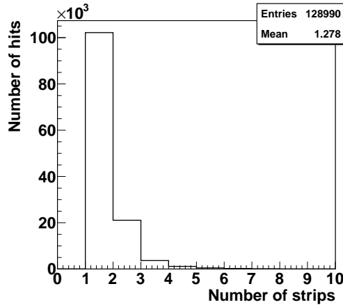
Рис. 3.11 Число стрипов в кластере, в эксперименте.
