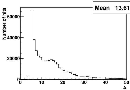
а) Рис. 3.12 Амплитуды сигнала до разделения кластеров
