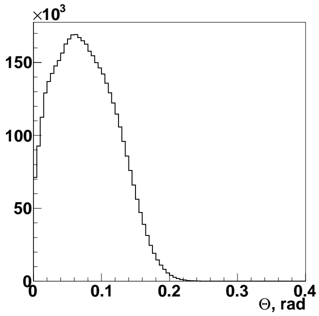
Рис. 3.38 Распределение треков в пространстве по полярному углу \Theta .
