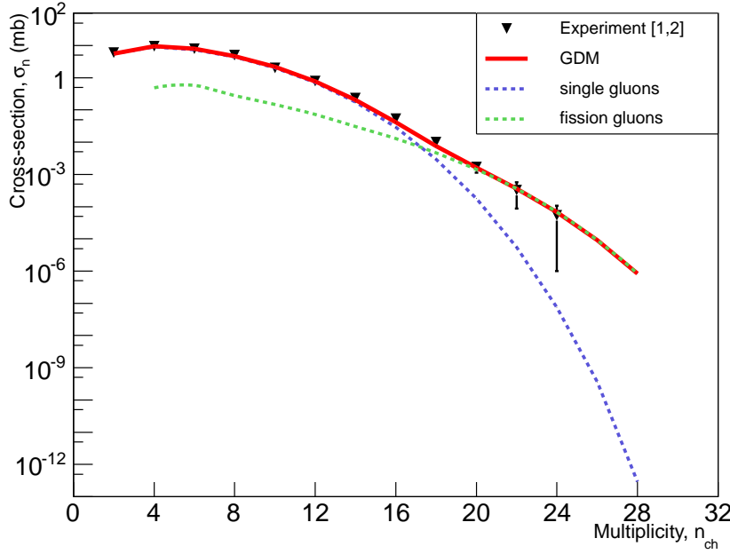
Рис. 5.7 Топологические сечения \sigma_n для pp соударений при 50 ГэВ с учётом ветвления.
