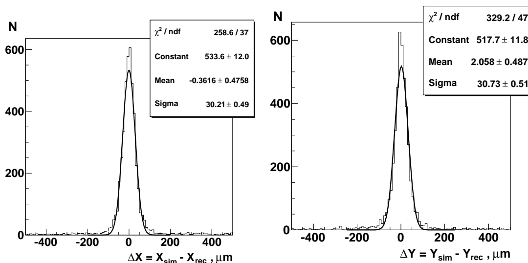
Рис. 3.33 Распределения по координатам X и Y вершин для моделированных событий.
