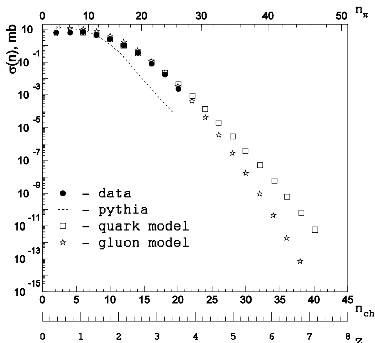
Рис. 1 Сравнение топологических значений \sigma(n_{ch}) для pp - взаимодействий при 70 ГэВ с кварковой моделью, с глюонной моделью — (МГД) и Монте-Карло генератором событий РУТНІА.
