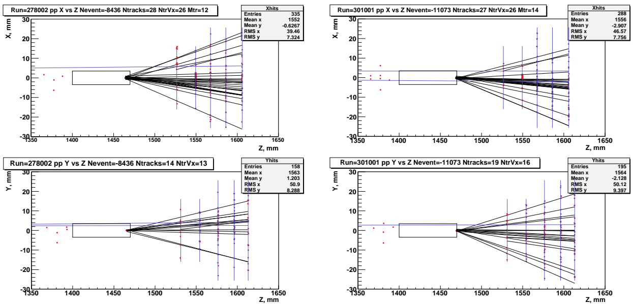
Рис. 4.33 Ложные события с множественностью 26 треков на X-проекции. Событие слева с Nch_x = 26 и Nch_y = 13 . Событие (справа) с Nch_x = 26 и Nch_y = 16 . Шумит середина второй плоскости на X-проекции (Gassiplex).
