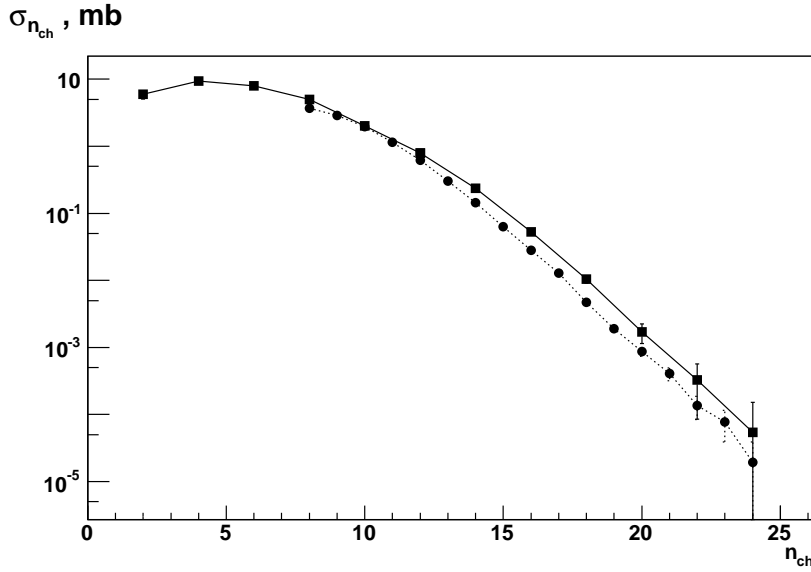
Рис. 5.4 Экспериментальные топологические сечения для pp -взаимодействия при 50 ГэВ перед и после введения поправок. Чёрные кружки — непоправленное распределение. Чёрные квадраты — поправленное распределение.
