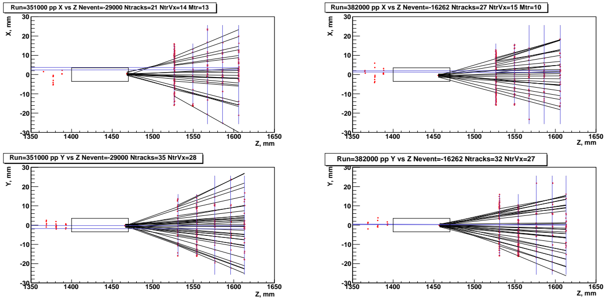
Рис. 4.32 Ложные события с множественность 27 и 28 треков на Y-проекции. Событие слева с Nch_x = 14 и Nch_y = 28 . Событие (справа) с Nch_x = 15 и Nch_y = 27 . Шумят первые две микростриповые плоскости (Gassiplex).
