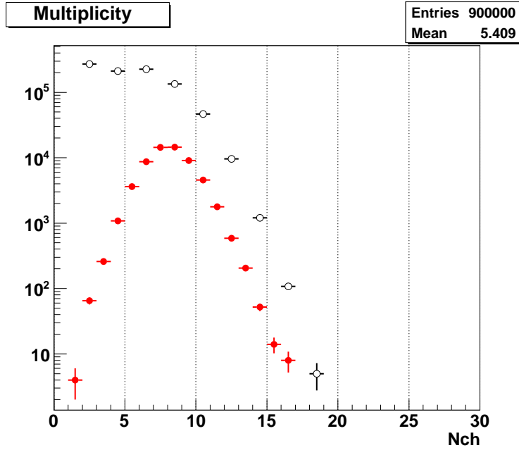
Рис. 5.1 Распределения по множественности. Белые кружки - генерированные события pythia для 52.5 ГэВ, красные кружки - реконструированные события в ВД с учётом триггера на 8 частиц.
