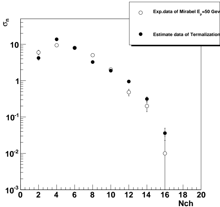
Рис. 5.2 Распределение по множественности для сечений с учётом эффективностей (чёрные кружки) и для сечений данных 'Мирабели' (белые кружки).
