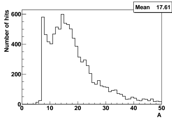
б) Рис. 3.13 Амплитуды сигнала после разделения кластеров
